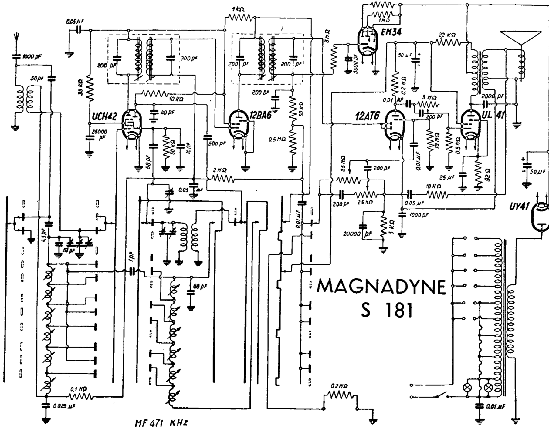
MAGNADYNE RADIO - Mod. S 181. Una gamma onde medie e sei bande allargate a onde corte (49, 41, 31, 25, 19 e 16 m.). Media frequenza 471 kc/s. Controllo di volume con compensazione dei toni bassi, a reazione inversa.
